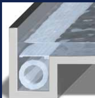
Couverture immergée – Compartiment au fond de la piscine
