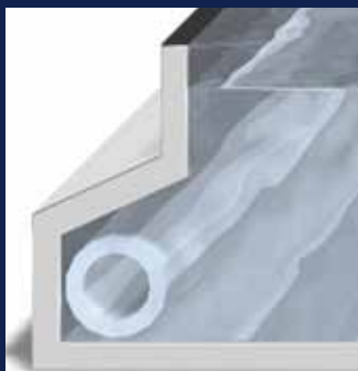
Instalación sumergida: Cajón en la prolongación del suelo del vaso
